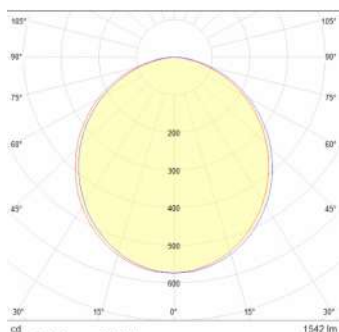
Unión X 100°
