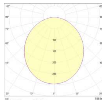
Unión L 100°
