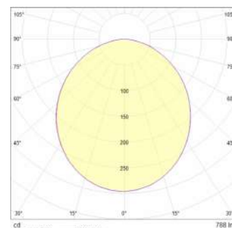
Unión L 100°
